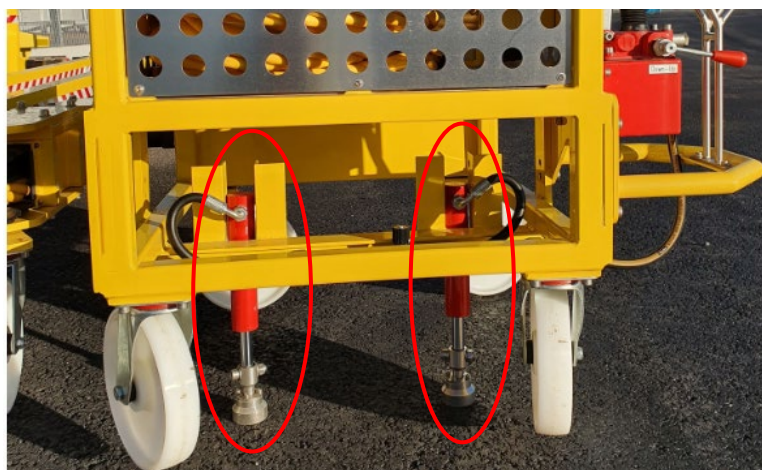
Stödben som lyfter kabelkorgen
