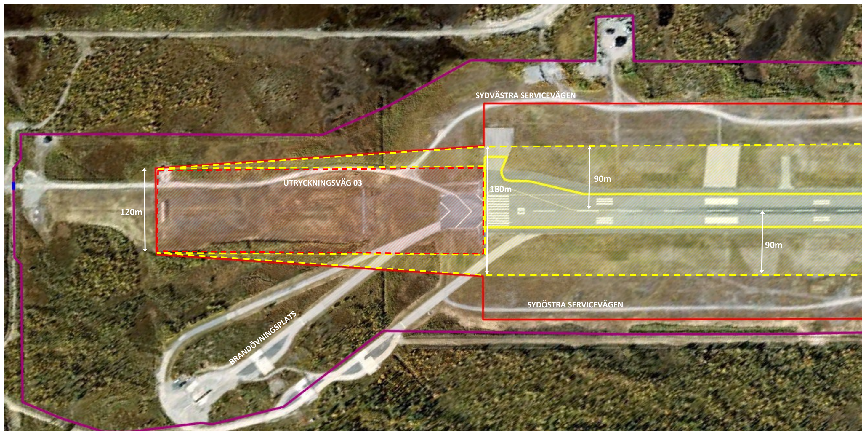
KARTA SKYDDSOMRÅDE ILS LLZ / CHART SAFETYAREA ILS LLZ KIRUNA AIRPORT
